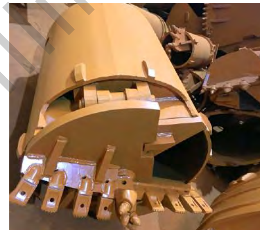
▲ 双底宝峨齿钻斗 Bottom bauer bucket
